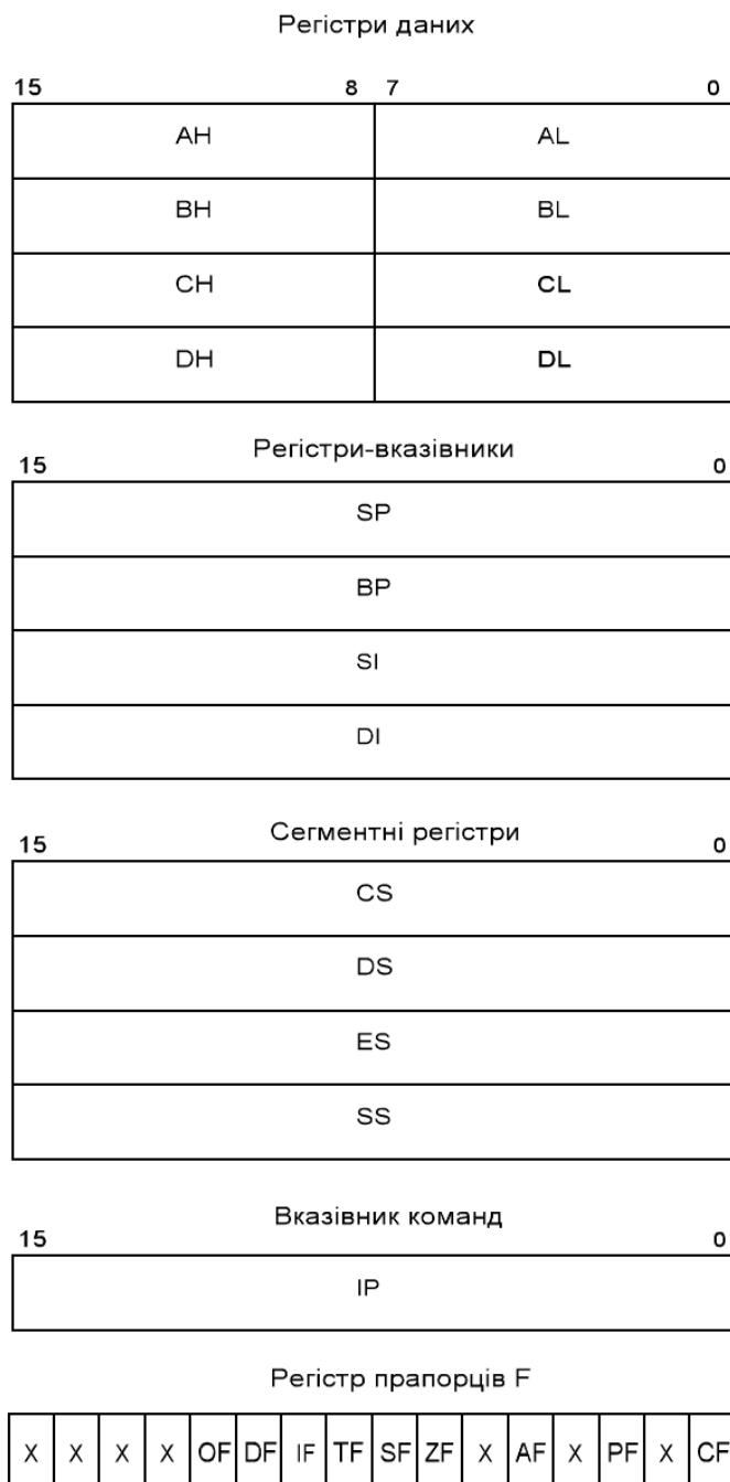
Рисунок 1 - Програмна модель МП i8086
